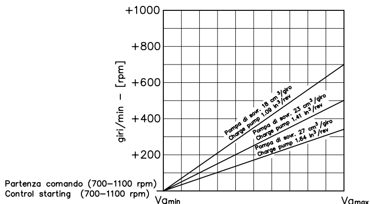
CURVA REGOLAZIONE CILINDRATA DISPLACEMENT VARIATION CURVES
