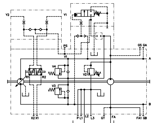
HIN con valvole di taglio
